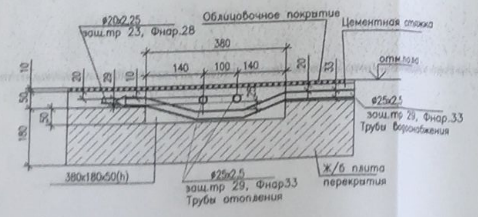
Разрез 1-1
